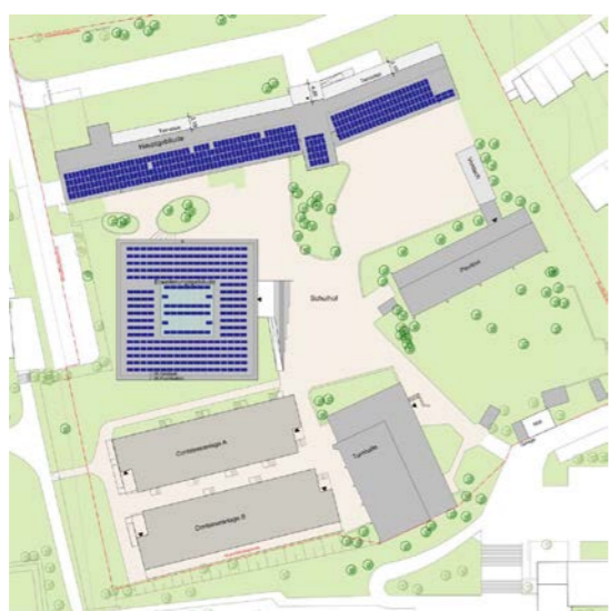
Lageplan
